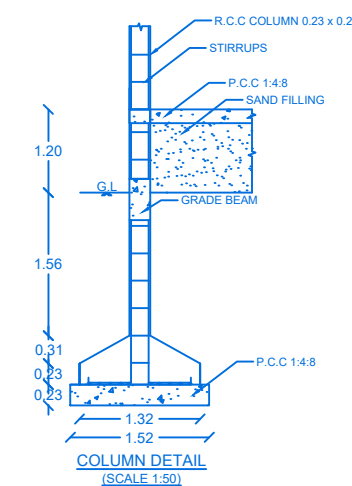
COLUMN DET (SCALE 1:50)
