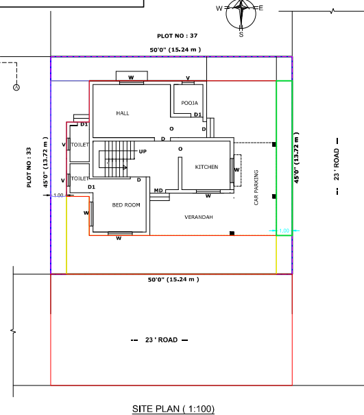
SITE PLAN ( 1:100)
