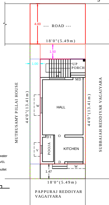
SITE PLAN ( 1:100)
