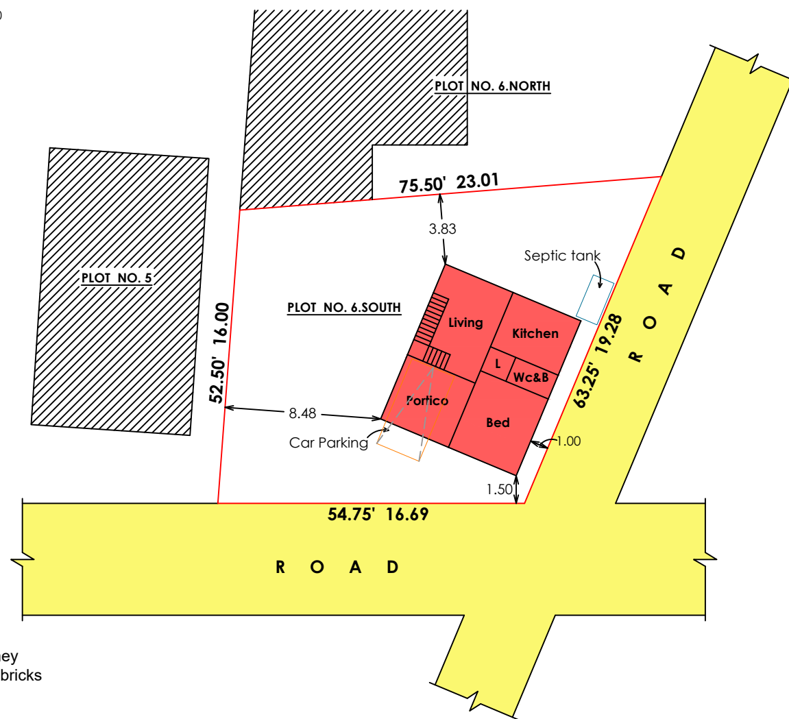
SITE PLAN SCALE - 1:250
