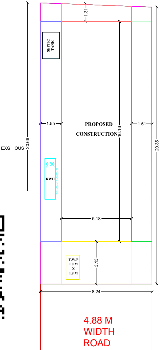
SITE PLAN SCALE : 1"= 8' OR [1 : 100]
