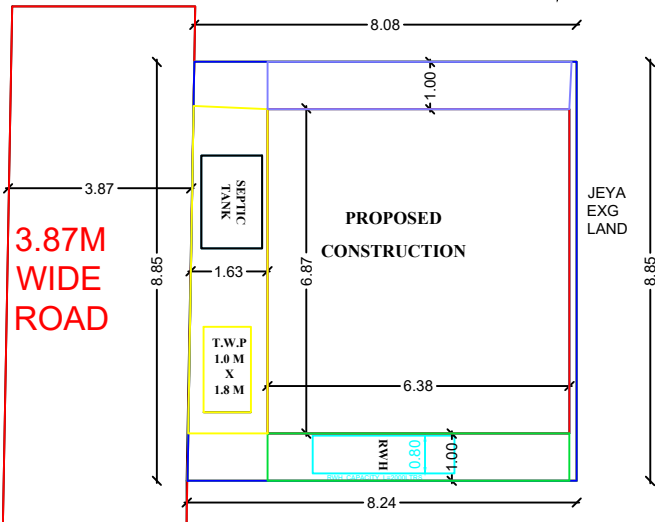
SITE PLAN SCALE : 1"= 8' OR [ 1 : 100]
