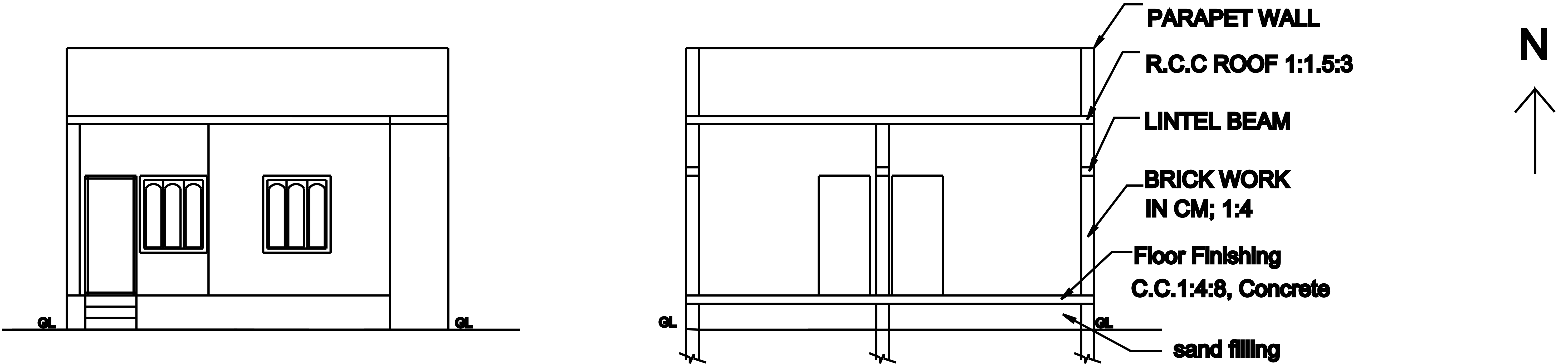
ELEVATION
