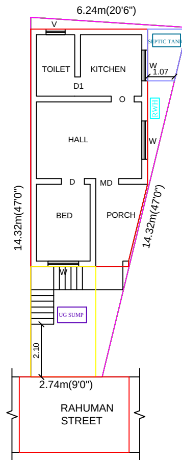
SITE PLAN SCALE 1:100
