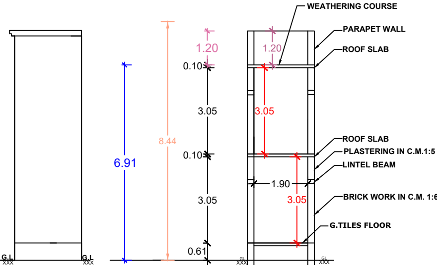
ELEVATION
