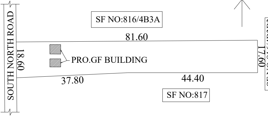
SITE PLAN (NTS)
