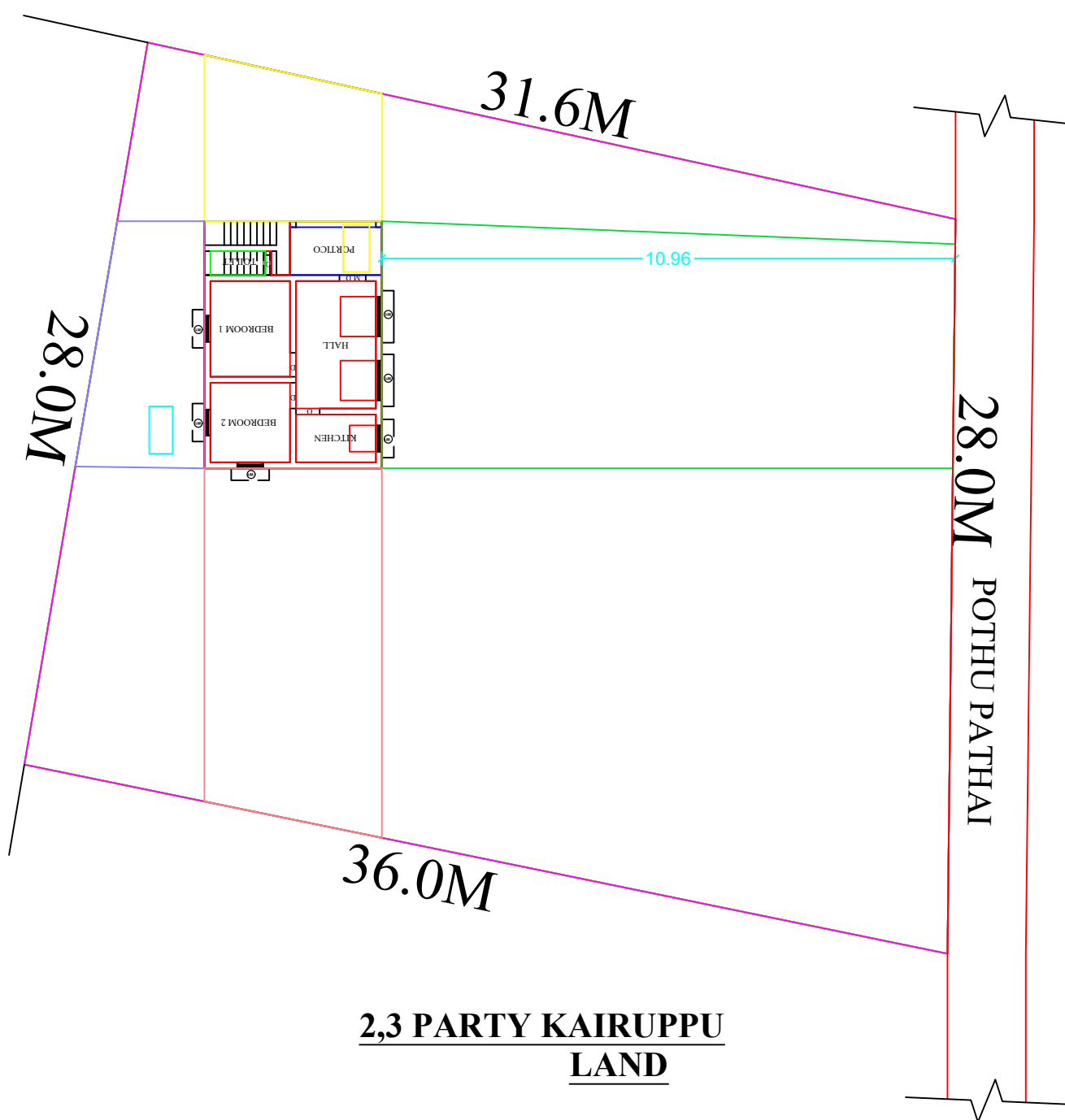
SITE PLAN(1:200)
