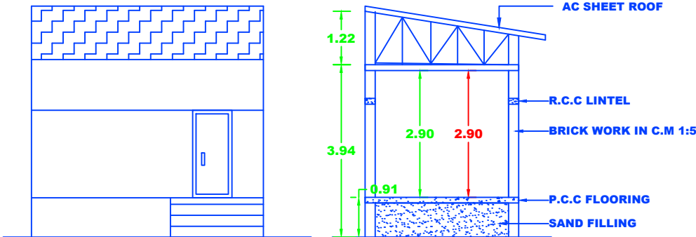
ELEVATION
