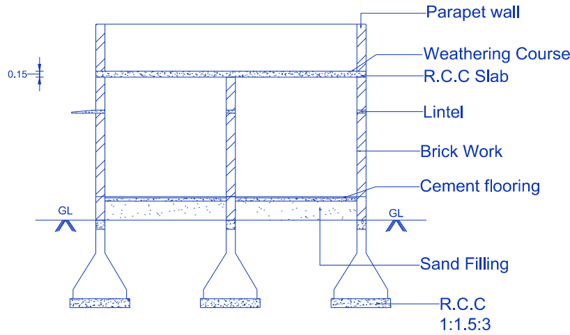
SECTION ON'AB'
