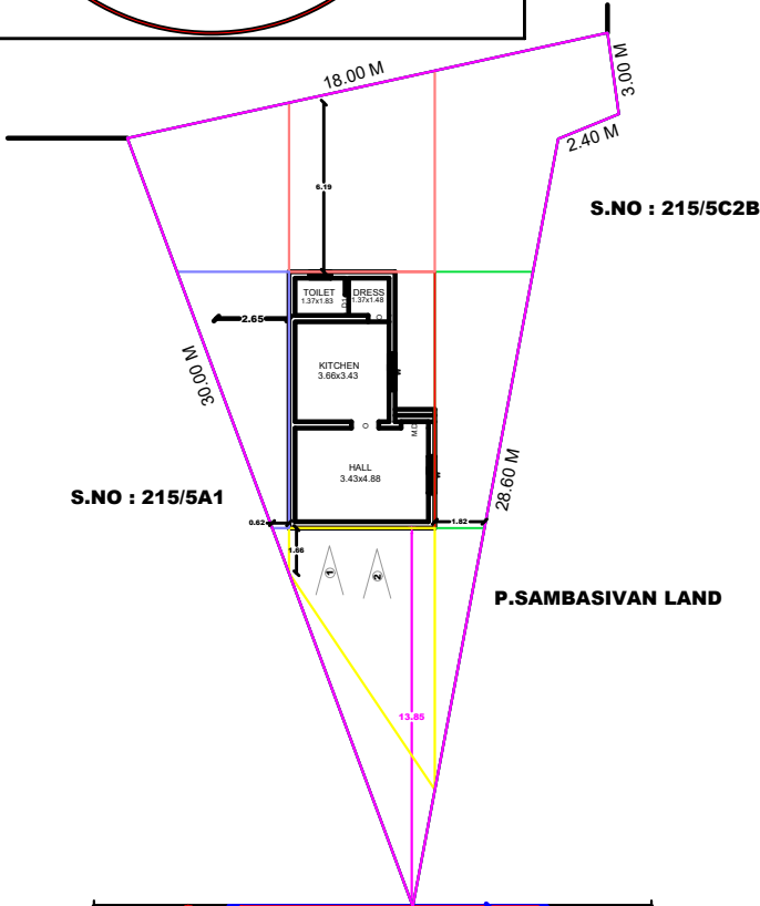
TOPO PLAN SCALE N.T.S
