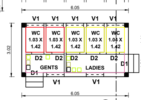
PLAN TOILET
