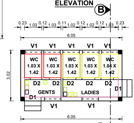
ELEVATION B
