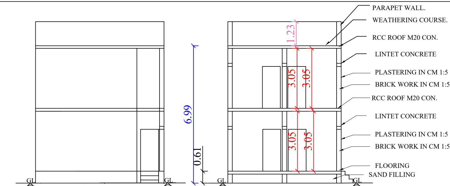
ELEVATION
