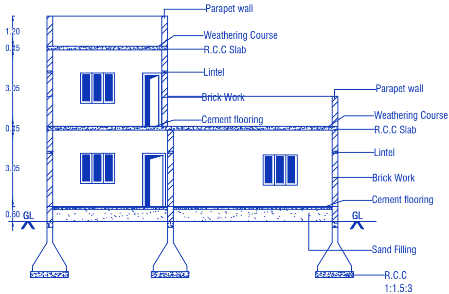
SECTION ON'AB'
