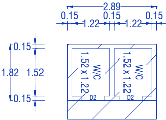
TOILET PLAN
