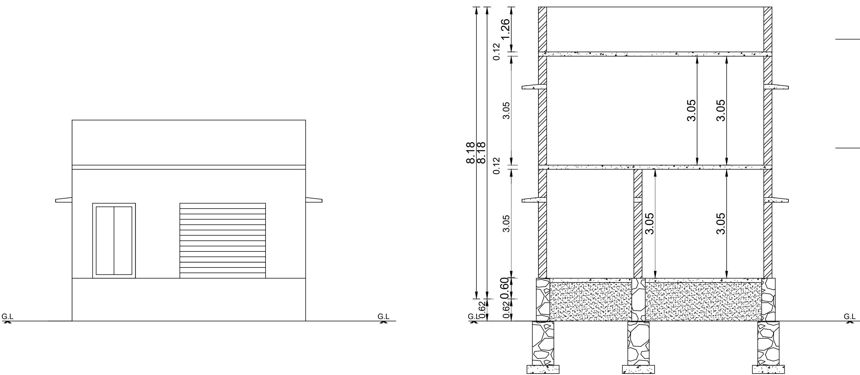
ELEVATION
