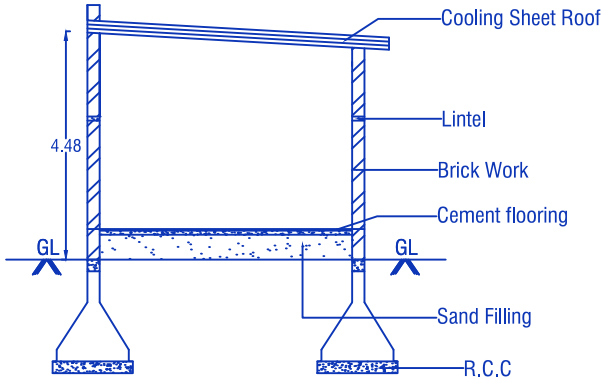
SECTION ON'AB'
