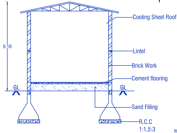
SECTION ON'AB'
