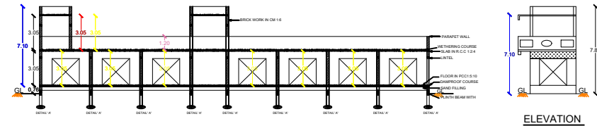
SECTION A-A
