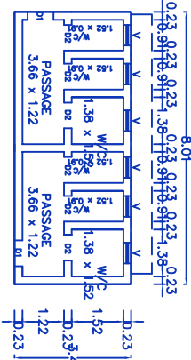
TOILET PLAN
