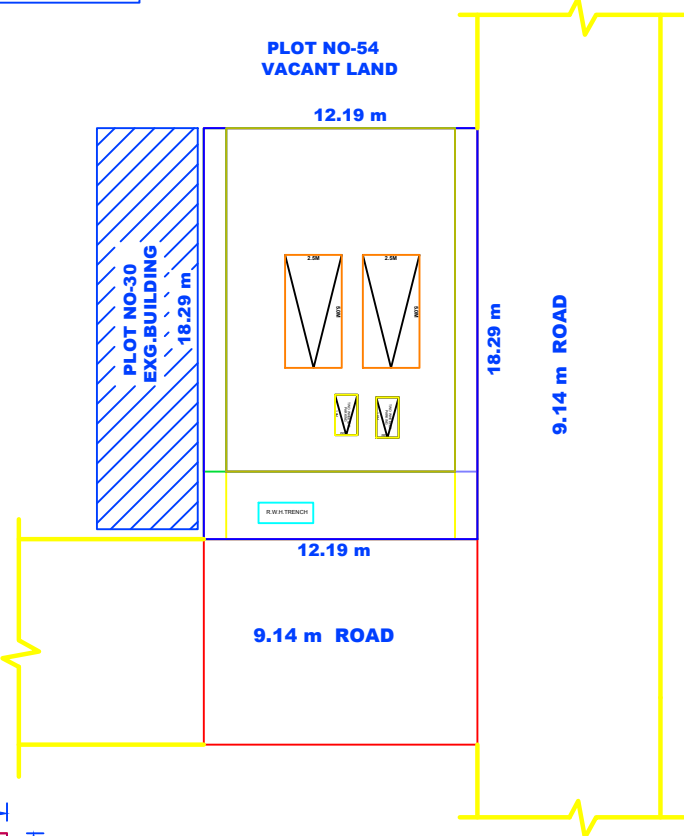
SITE PLAN 1:200
