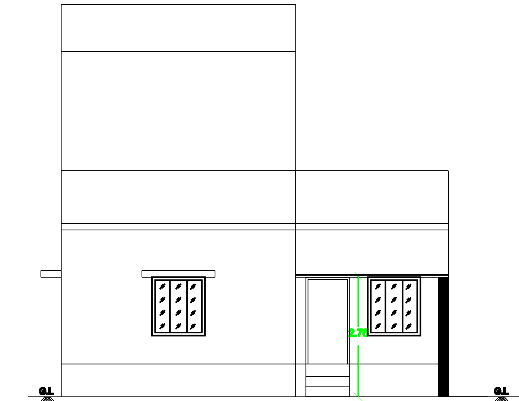
ELEVATION
