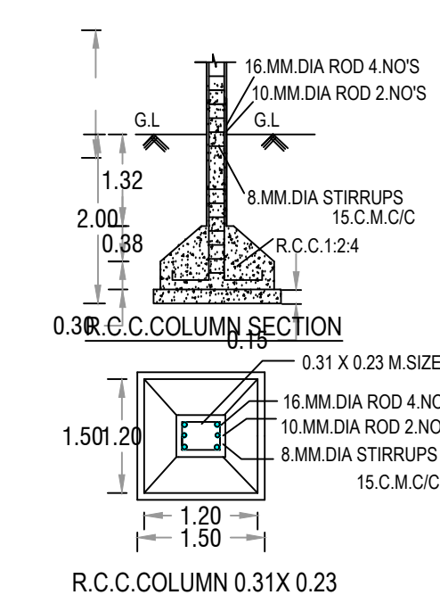
R.C.C.COLUMN 0.31X 0.23
