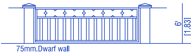
ELEVATION
