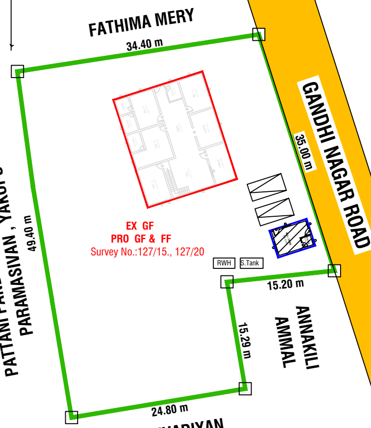
SITE PLAN (1:300)
