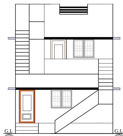
ELEVATION
