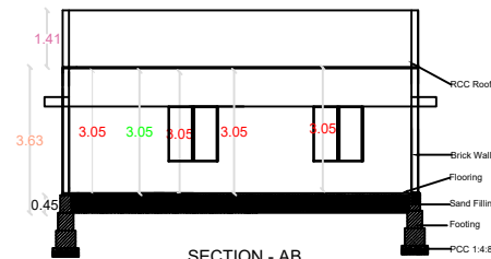
SECTION - AB
