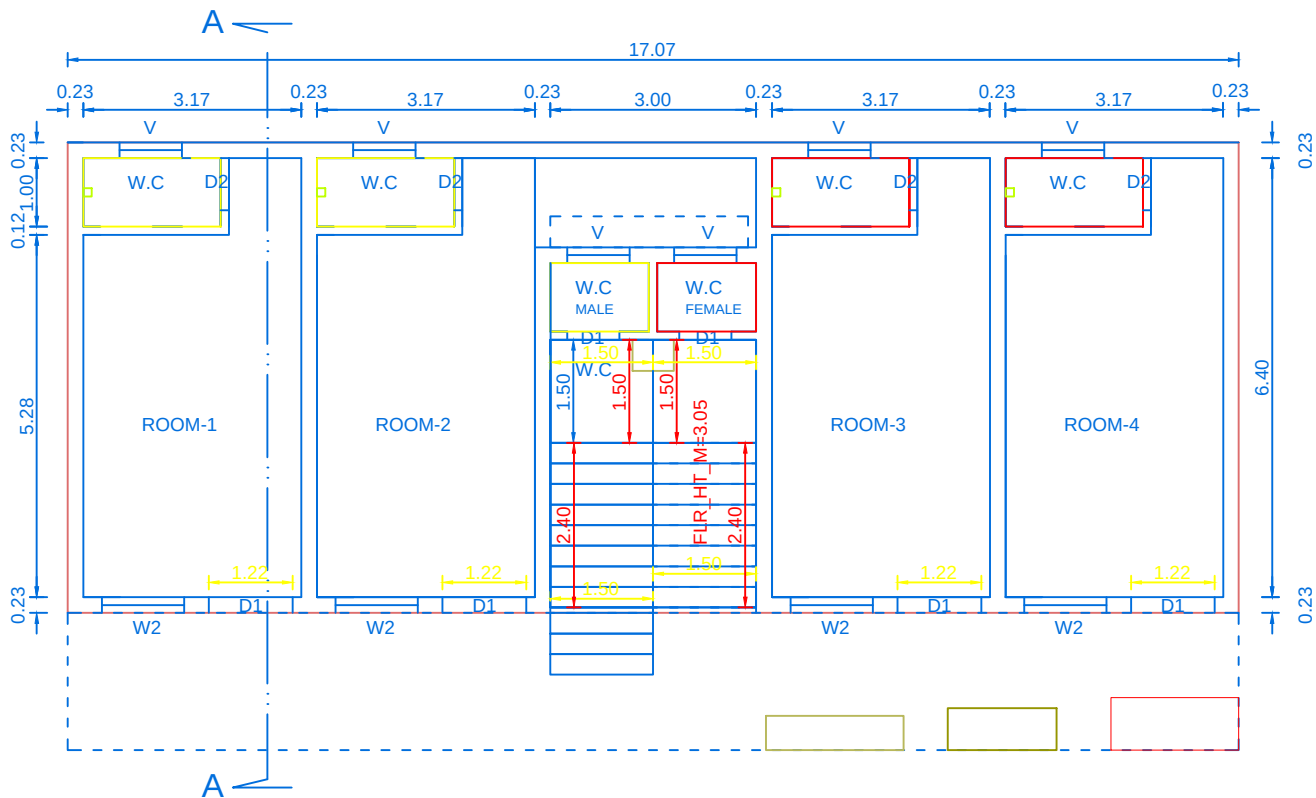
PROP.FIRST FLOOR
