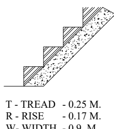
STAIRCASE DETAILS - N.T.S
