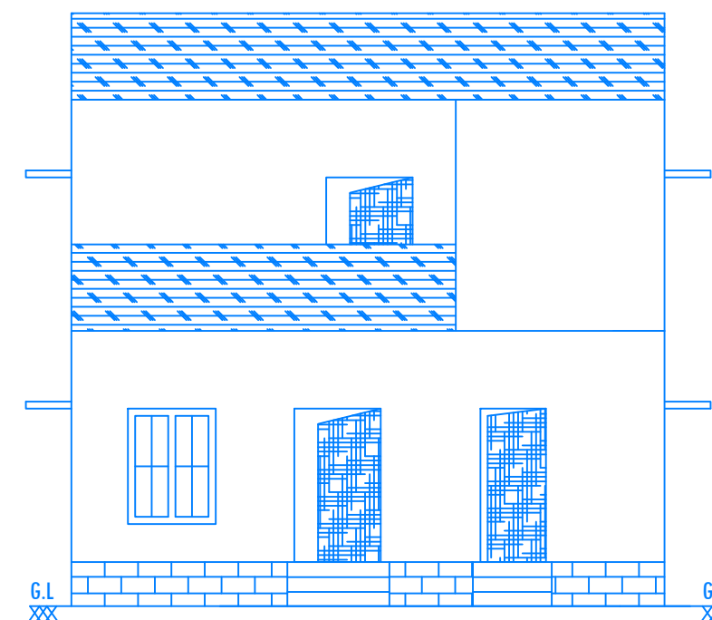
ELEVATION
