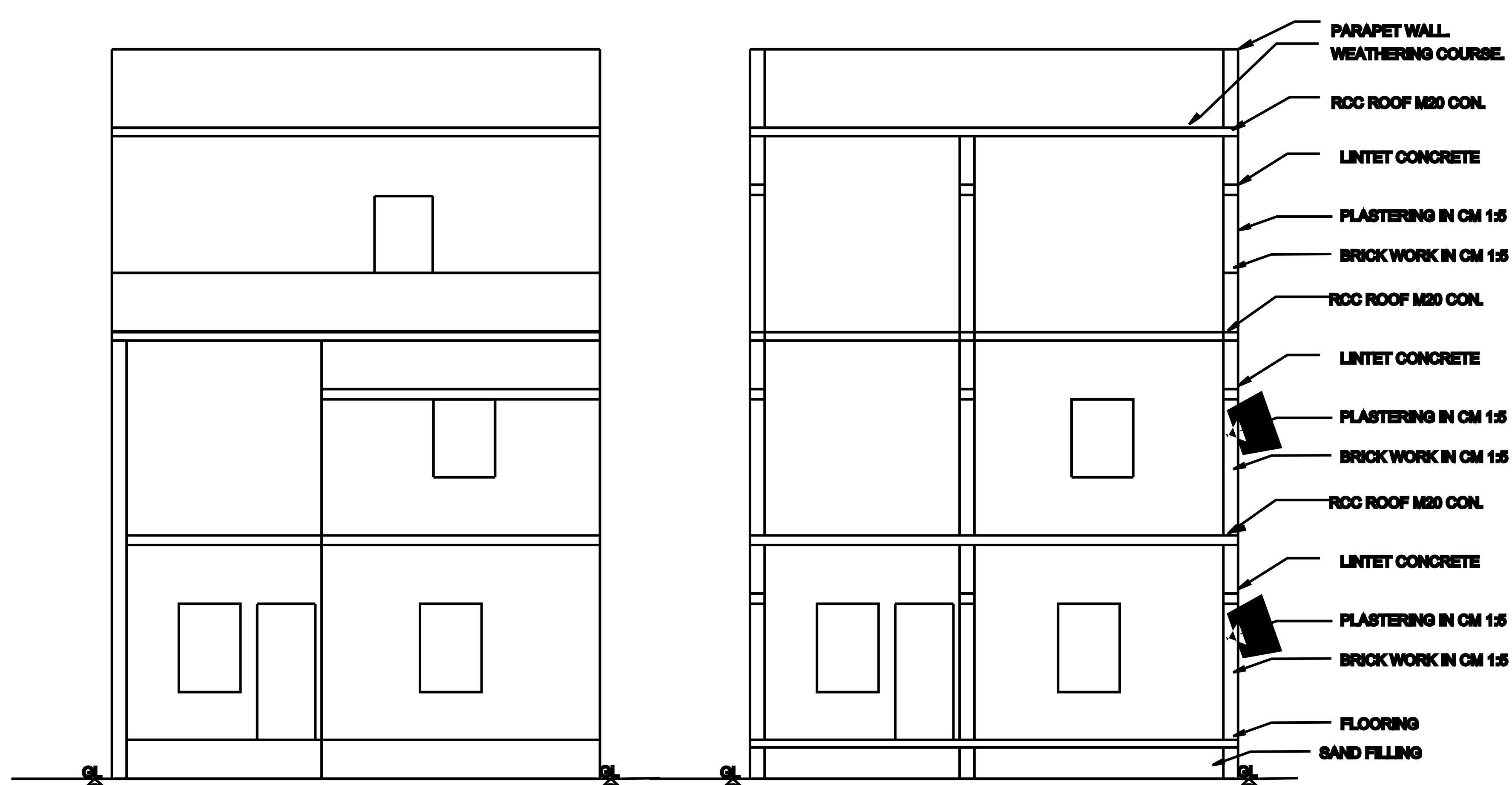
ELEVATION
