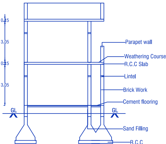
SECTION ON'AB'
