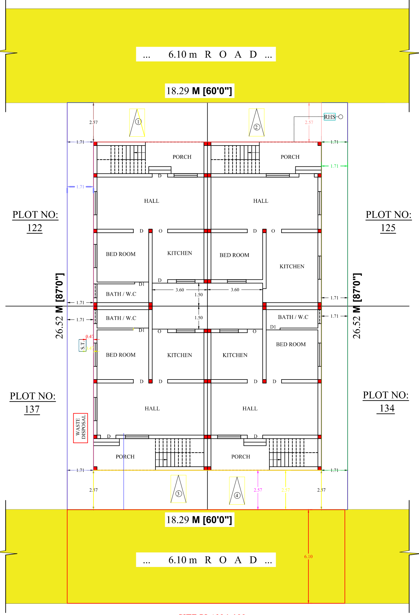
SITE PLAN 1:100
