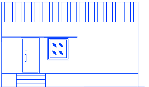
ELEVATION
