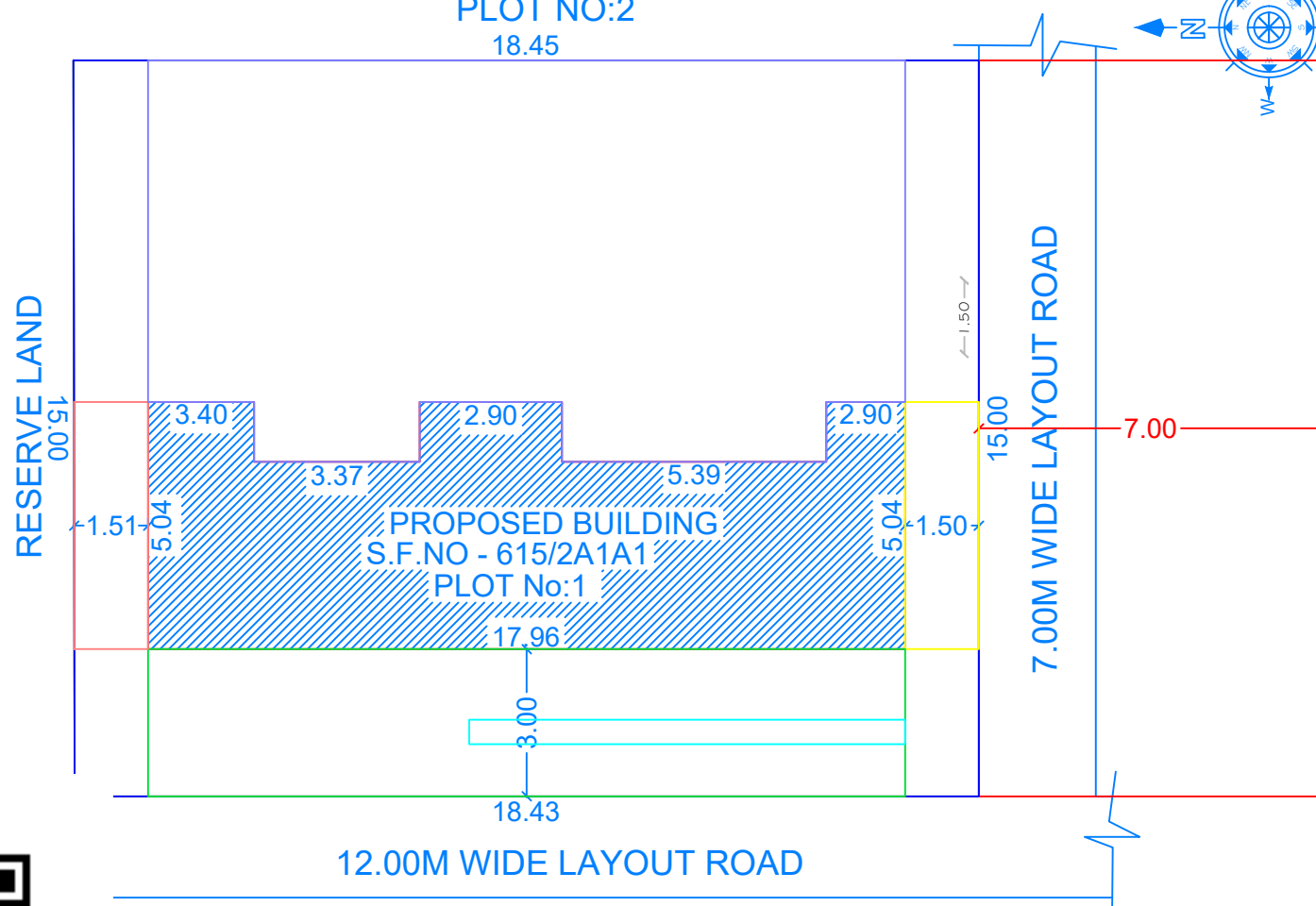
SITE PLAN 1:100
