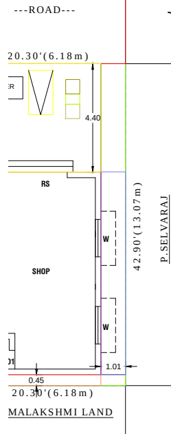
SITE PLAN (SCALE : - 1:100)
