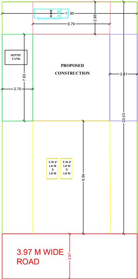
SITE PLAN SCALE : 1"= 8' OR [1 : 100]
