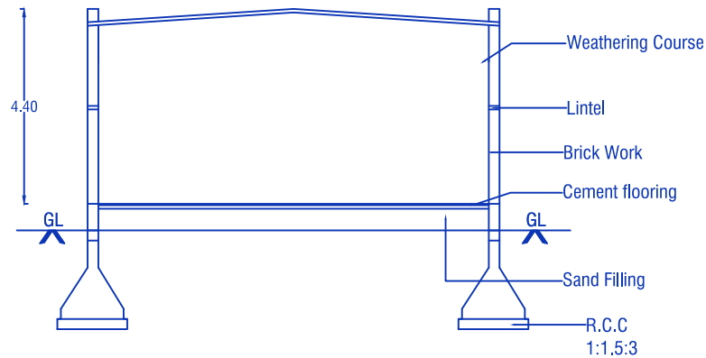
SECTION ON'AB'
