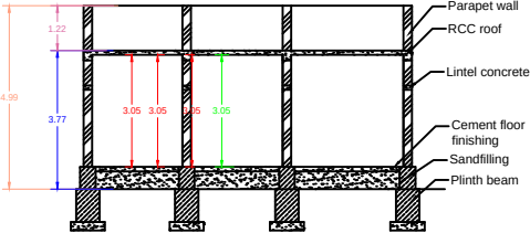
SECTION - AB
