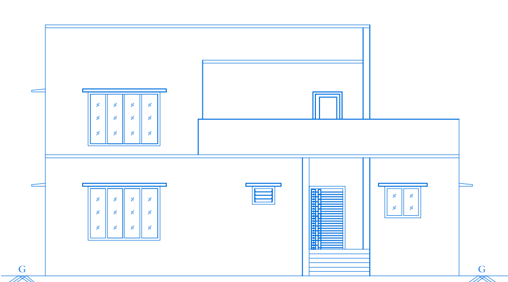
ELEVATION
