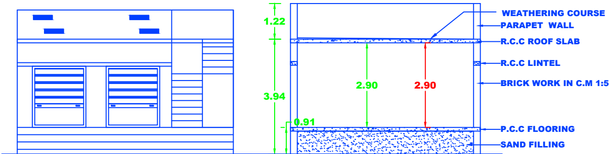
ELEVATION
