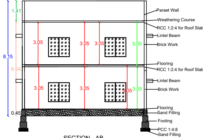
SECTION - AB
