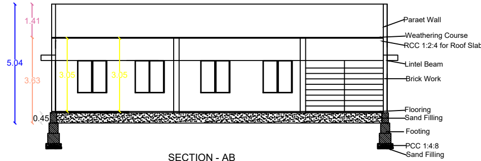
SECTION - AB
