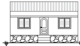
ELEVATION-A
