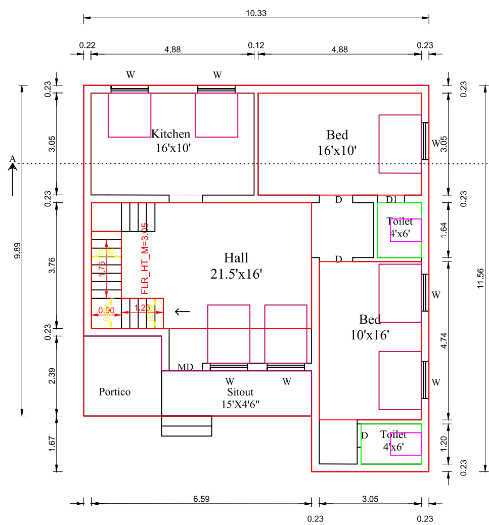
G.F PLAN
