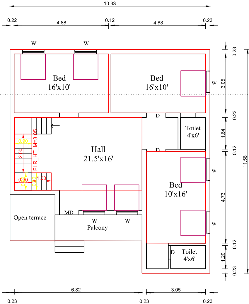
F.F PLAN
