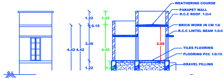
ELEV
