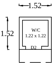
TOILET PLAN
